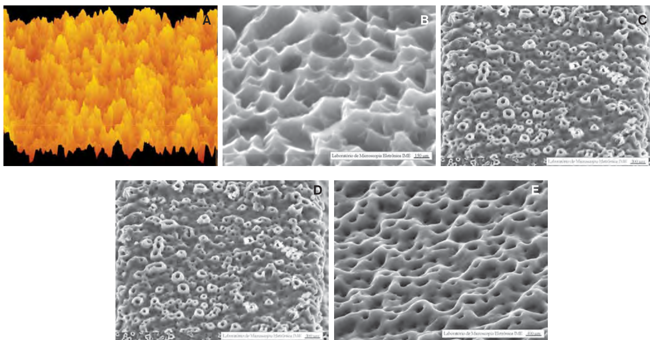
Figura 3a, 3b, 3c, 3d e 3e (A e B) Superfície do implante comercial Master Porous tratado com ácido; (C) Superfície tratada com jateamento de óxido de titânio; (D) Superfície TiUnite anodizada; (E) Superfície Vulcano Actives.
